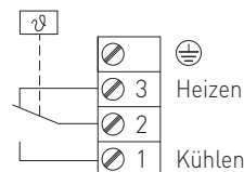
Anschlussbild
