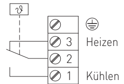
Anschlussbild
