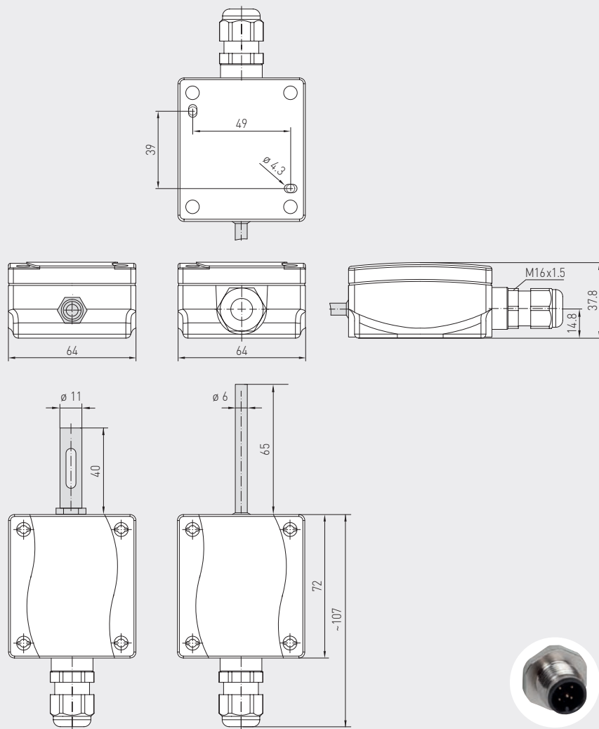
Габаритный чертеж
