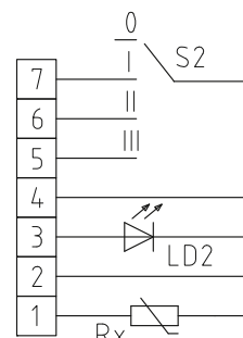
Схема соединения
