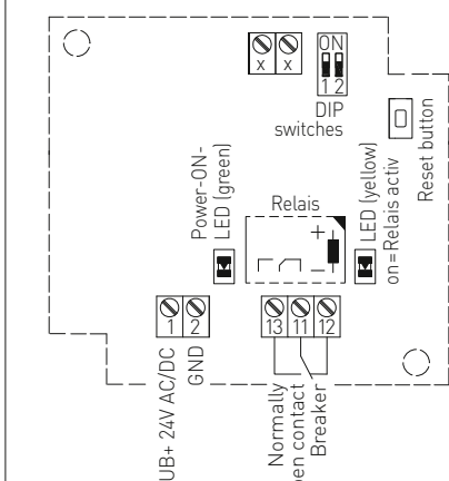
Схема подключения
