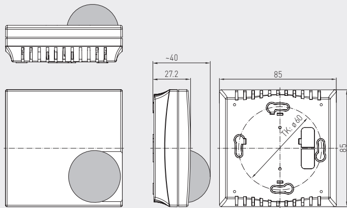
Габаритный чертёж
