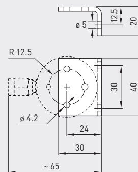
Габаритный чертеж [мм]
