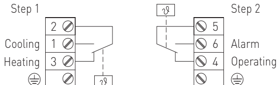
Схема соединения KTR TR + STB (двухступенчатый)
