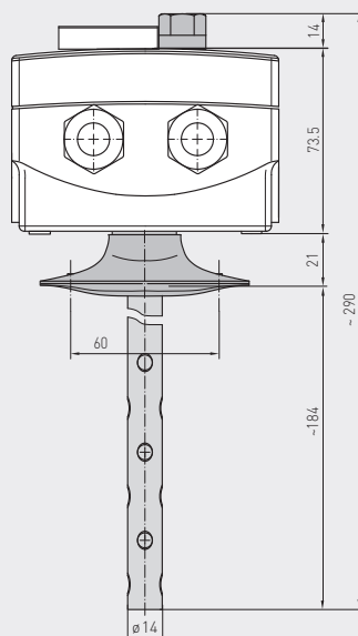
Габаритный чертеж Терморегулятор + регулируемый предохранительный ограничитель температуры TR + STB
