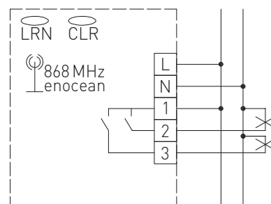
Схема подключения
