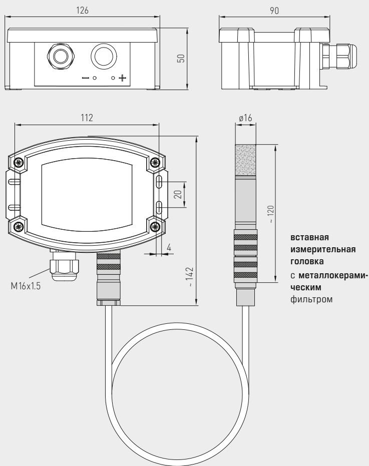
Габаритный чертеж
