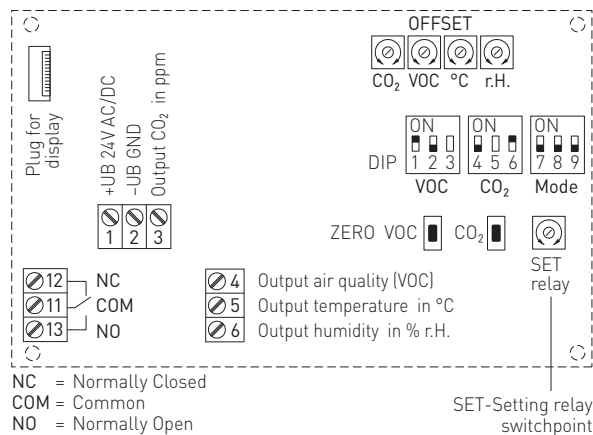
Схема подключения
