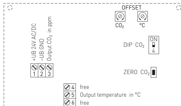
Схема подключения
