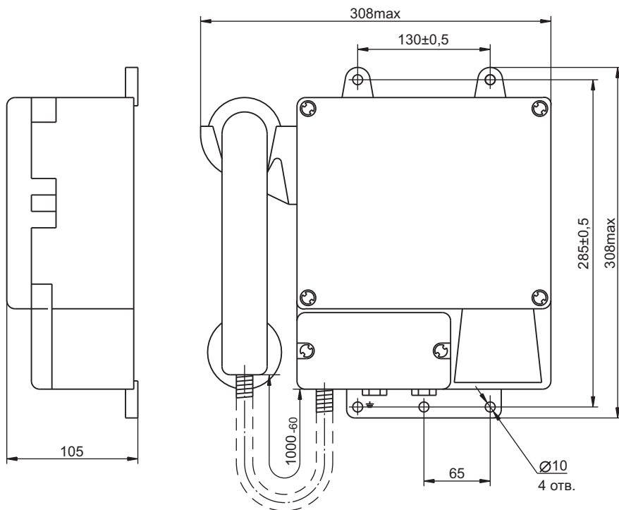
Рисунок 1. Аппарат телефонный шахтный ТАШ-2305
