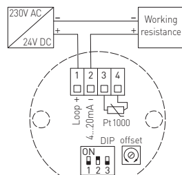
Schéma de raccordement RGTM 1-I
