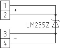
1х четырехпроводное подключение LM 235 Z (KP 10)
