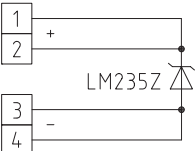
1x Vierleiterschaltung LM235Z (KP10)
