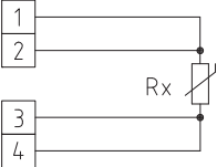
1x Vierleiterschaltung Standard
