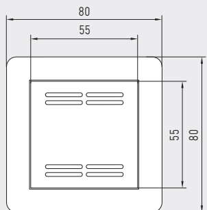
Габаритный чертёж [мм]
