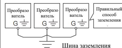
Рис. 1-1 (подключение к одной точке)
