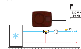
Схема 2 - управление подачей - охлаждение
