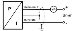
2-проводная линия (вых. сигнал - ток)
