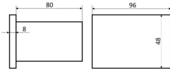
Габаритные размеры корпуса
