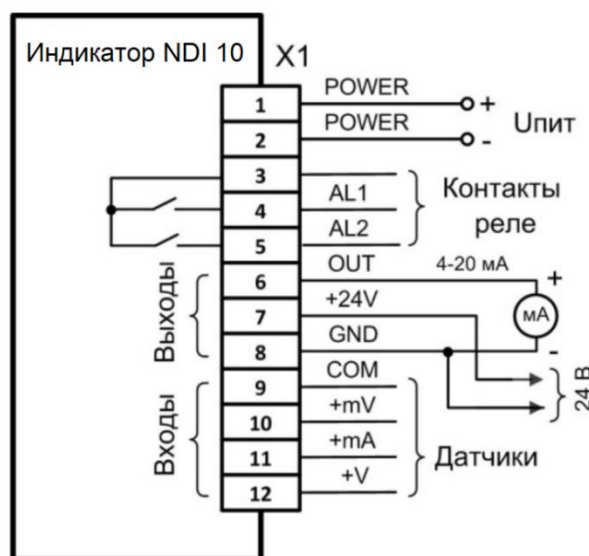
Схема подключения и контакты разъема
