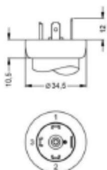
Код 100 или E00 (Разъем DIN 43650 (ISO 4400) / IP 65 или разъем DIN 43650 (ISO 4400) / IP 67)
