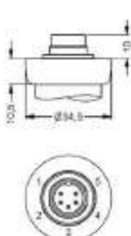
Код 200 (Разъем Binder 723, 5-конт. / IP 67)
