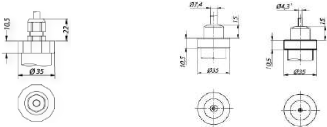
Код 400 (Каб. ввод PG7 с кабелем PVC 2 м / IP 67)
