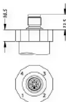
Код M00 или M10 (Разъ- ем M12x1, 4-конт. / IP 67 или разъем M12x1 металлический, 4-конт. / IP 67)
