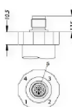
Код N00 или N10 (Разъ- ем M12x1, 5-конт. / IP 67 или разъем M12x1 металлический, 5-конт. / IP 67)
