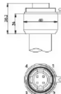
Код 500 (Разъем Bussanerg, 4-конт. / IP 68)
